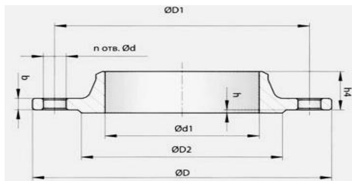
Фланец воротниковый ГОСТ 12821-80
